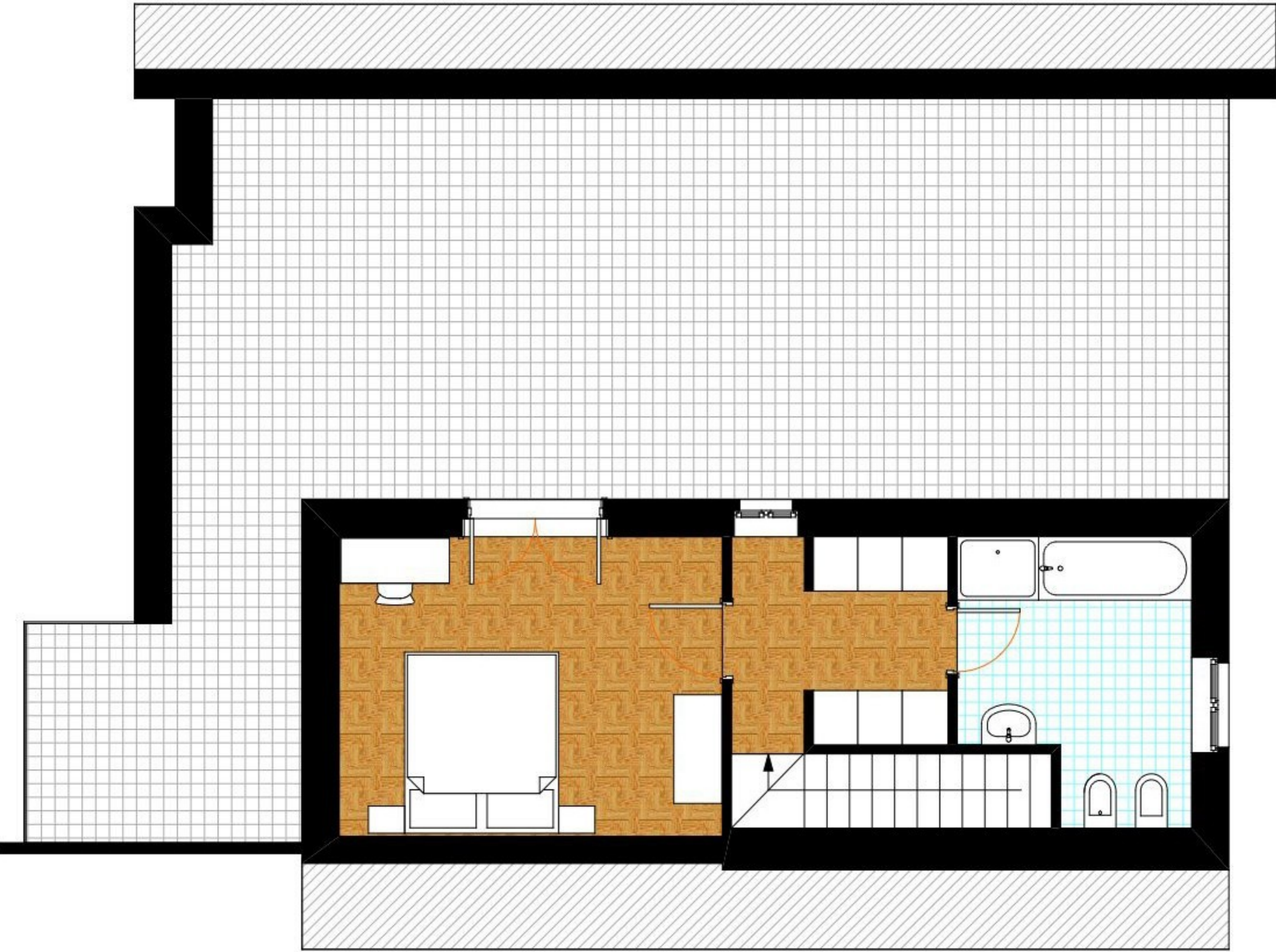
Unita' C40 - piano 4° sottotetto
